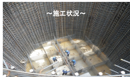
《3号橋P5橋脚_柱状体深礎基礎φ11m L=21m》
